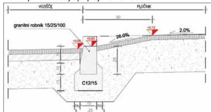
Prerez iz detajla po projektu Roške ceste
