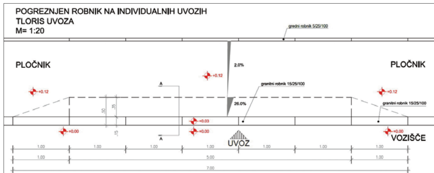
Tlorisni prikaz iz detajla po projektu Roške ceste
